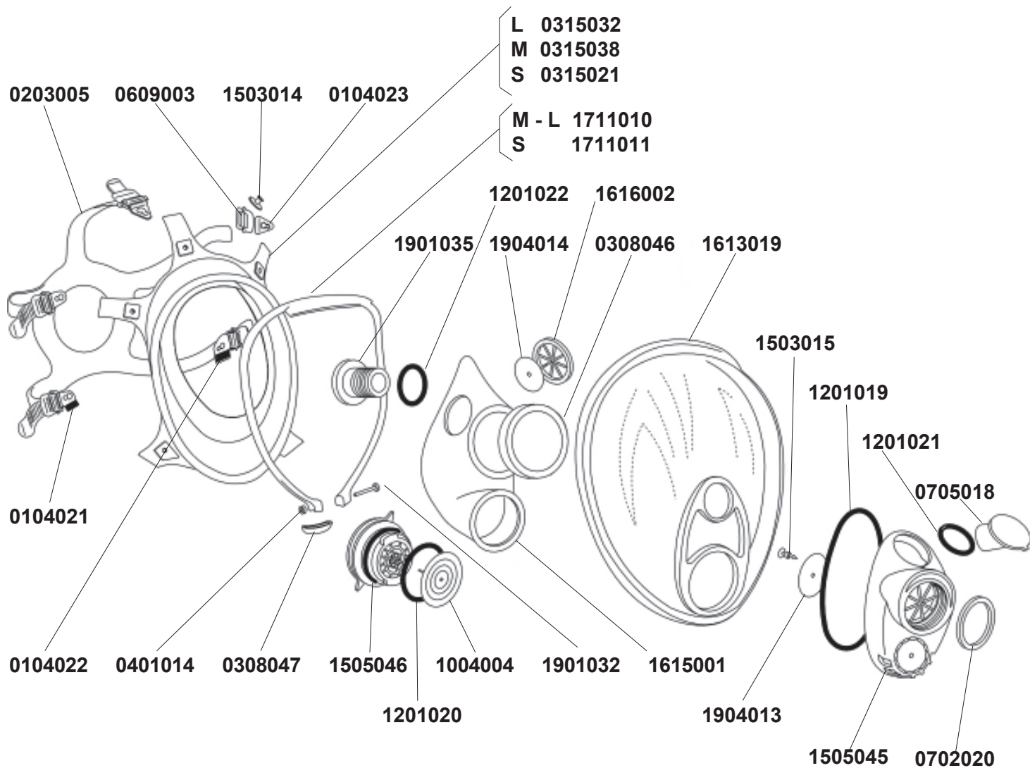
Centralina-Unit-Distributeur
